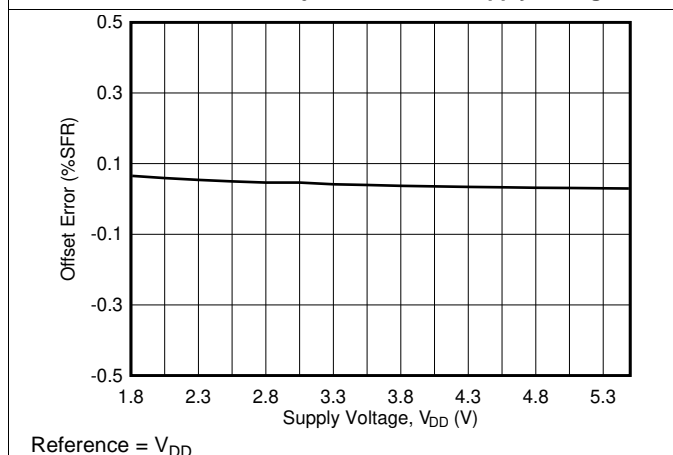
图 26. Offset Error vs Supply Voltage
