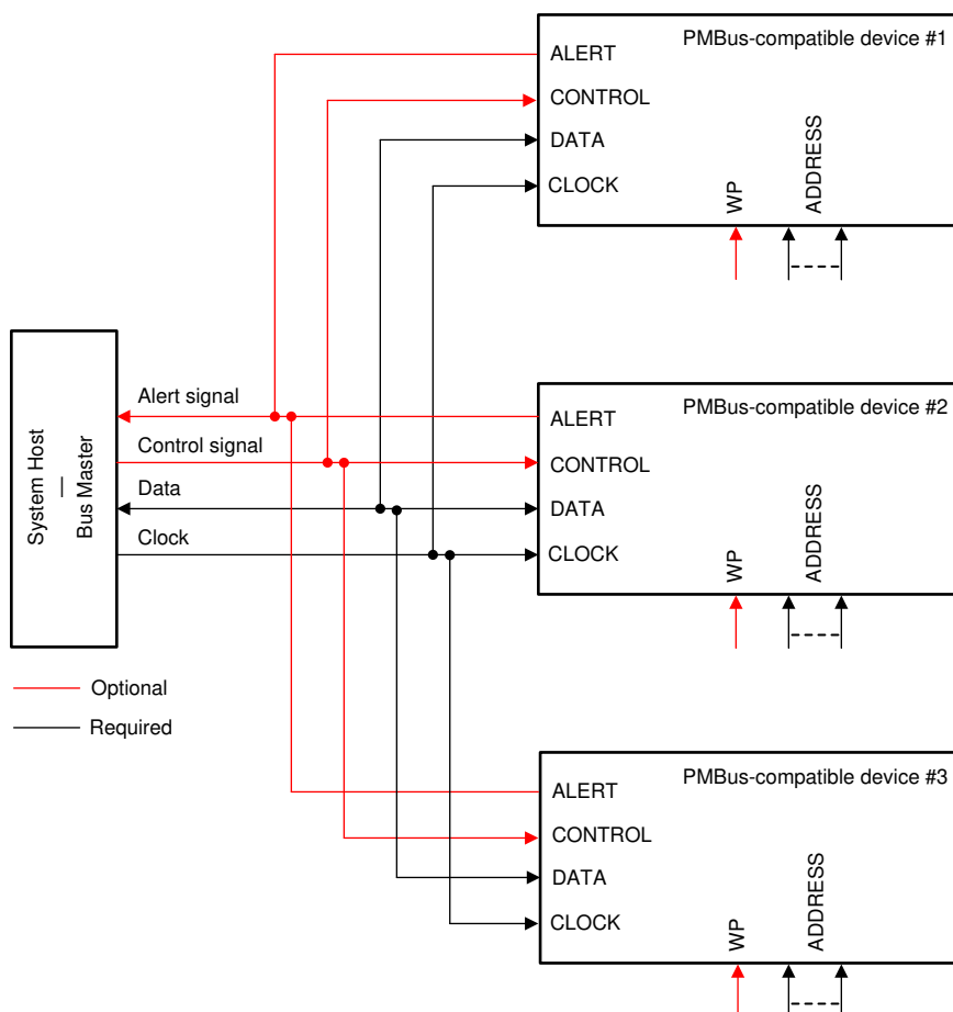
图 49. PMBus Connections
