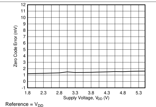
图 25. Zero-Code Error vs Supply Voltage
