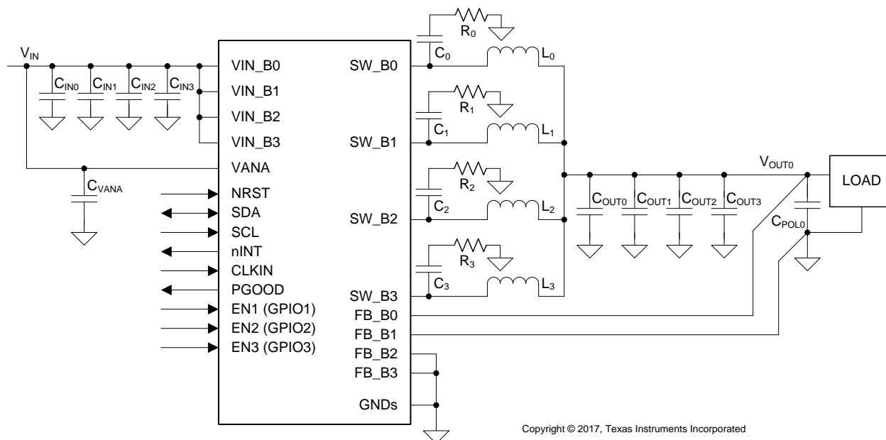
图 28. 4-Phase Configuration (LP87561-Q1)
