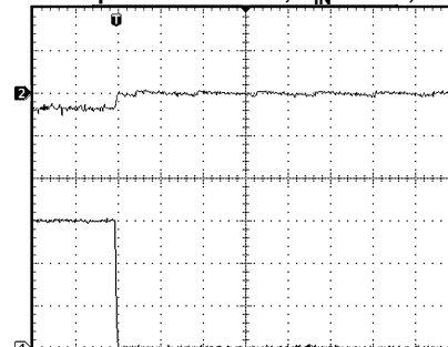
CH2: V_{OUT} ; Scale: 100mV/Div DC Coupled, Offset 1.834V CH4: I_{OUT} ; Scale: 100mA/Div Time scale: 4ms/Div
