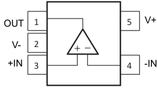
图 5-1. 5 引脚 SOT-23 DBV 封装 (LMV321A 顶视图)
