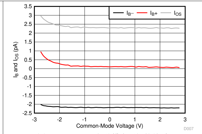
图 6-2. I_B 和 I_{OS} 与共模电压间的关系
