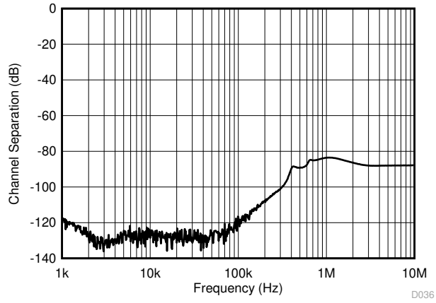
图 6-31. 通道分离
