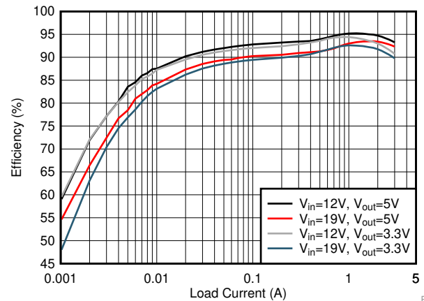
TPS56339 效率
