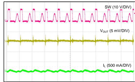
Time (2 \mu\text{s} /DIV)
