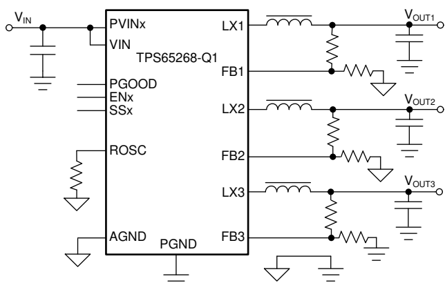
应用原理图
