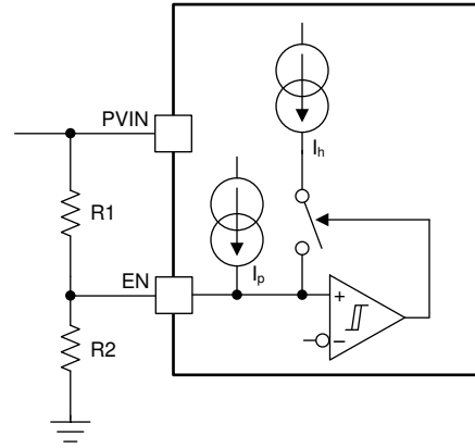
图 23. Adjustable PV_{IN} UVLO, V_{IN} > 4 V
