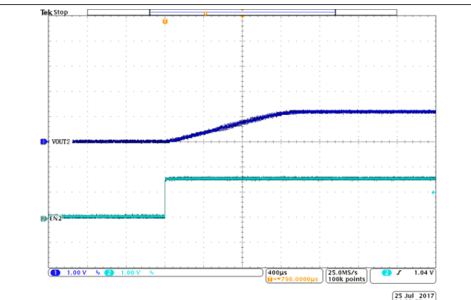
图 35. BUCK2 Soft-Start
