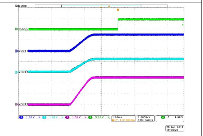
图 49. PGOOD
