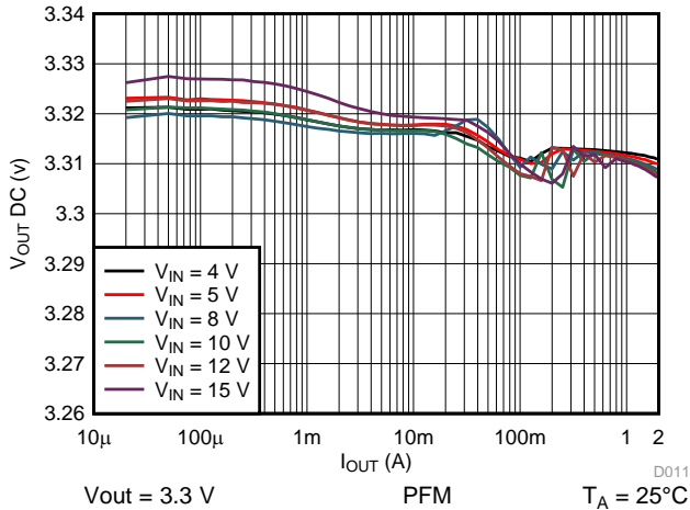
图 30. Output Voltage vs Output Current
