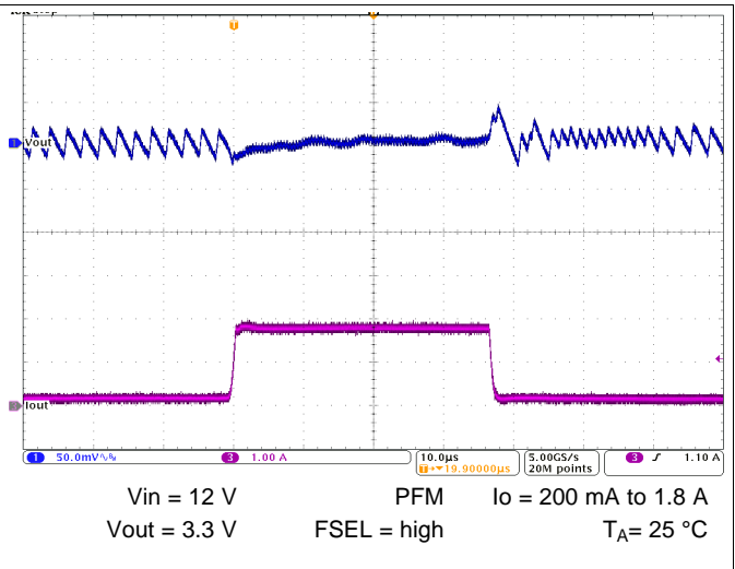
图 49. Load Transient Response
