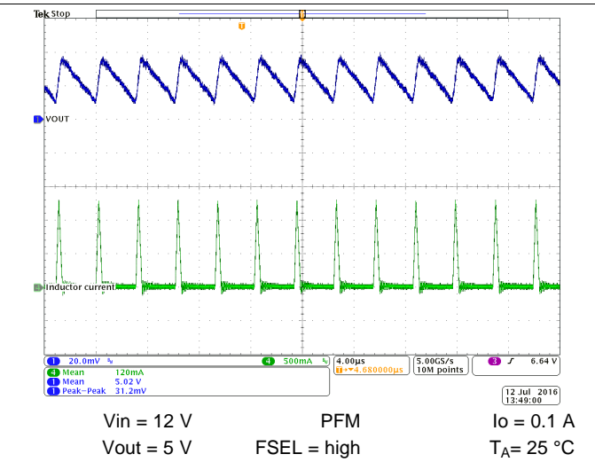
图 61. Output Voltage Ripple
