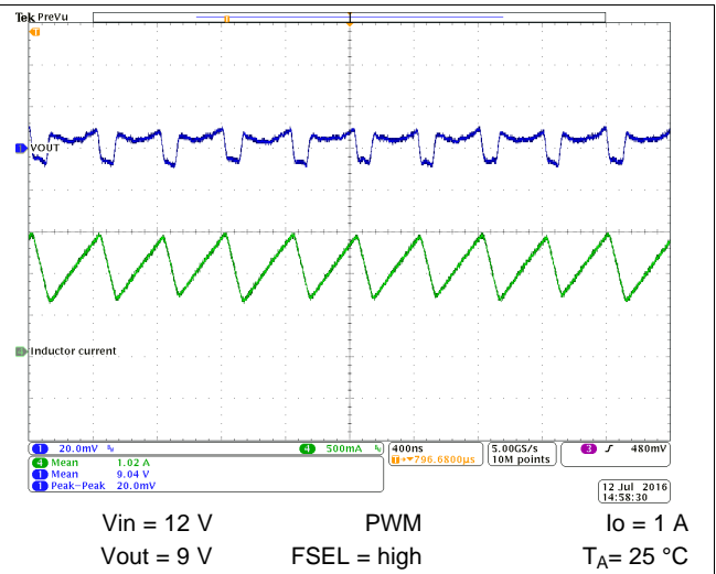
图 69. Output Voltage Ripple
