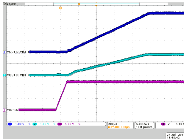
图 89. Tracking
