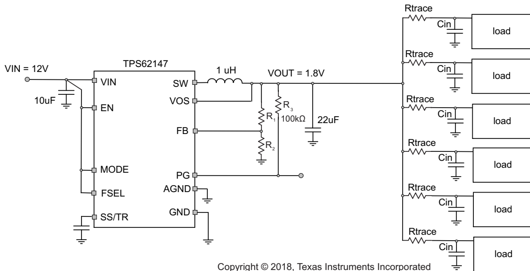
图 87. Multiple Loads
