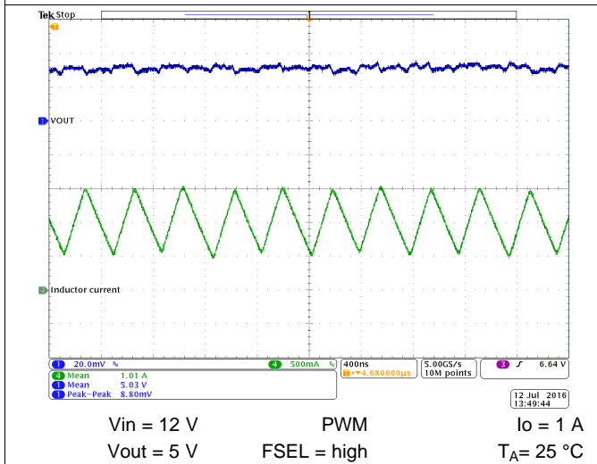
图 62. Output Voltage Ripple
