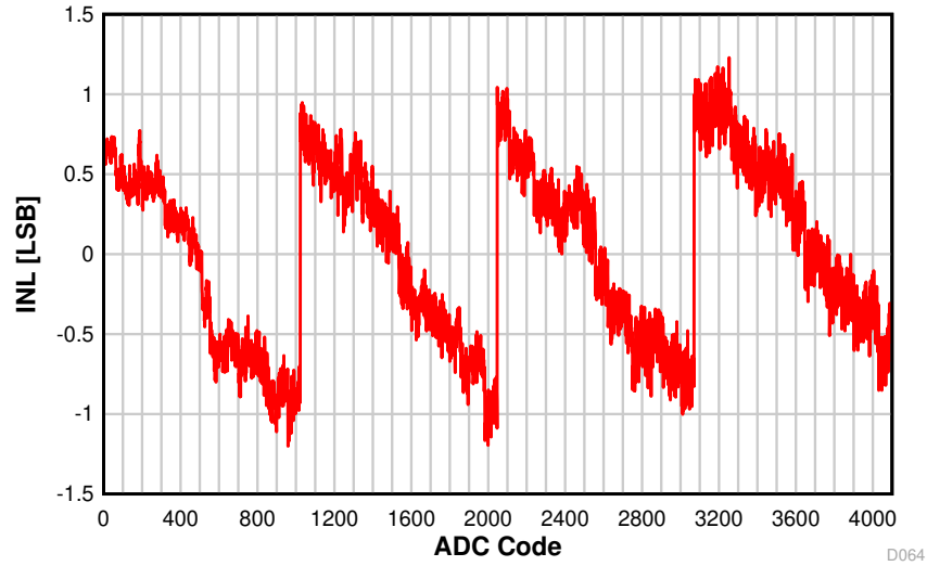
图 8-22. INL vs. ADC Code
