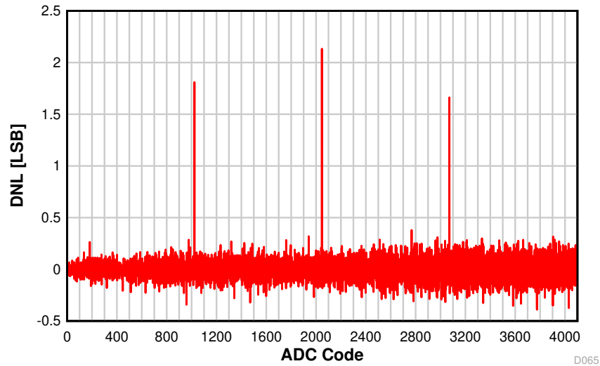
图 8-23. DNL vs. ADC Code
