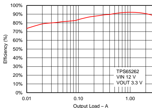
效率与输出负载之间的关系
