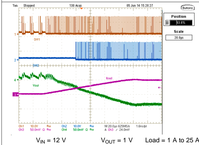
图 3. Load Transient
