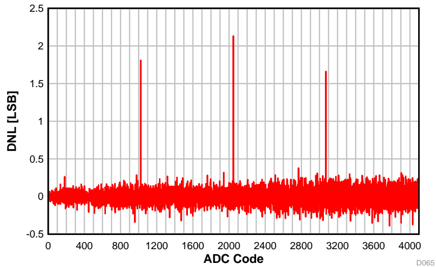
图 5-27. DNL vs. ADC Code
