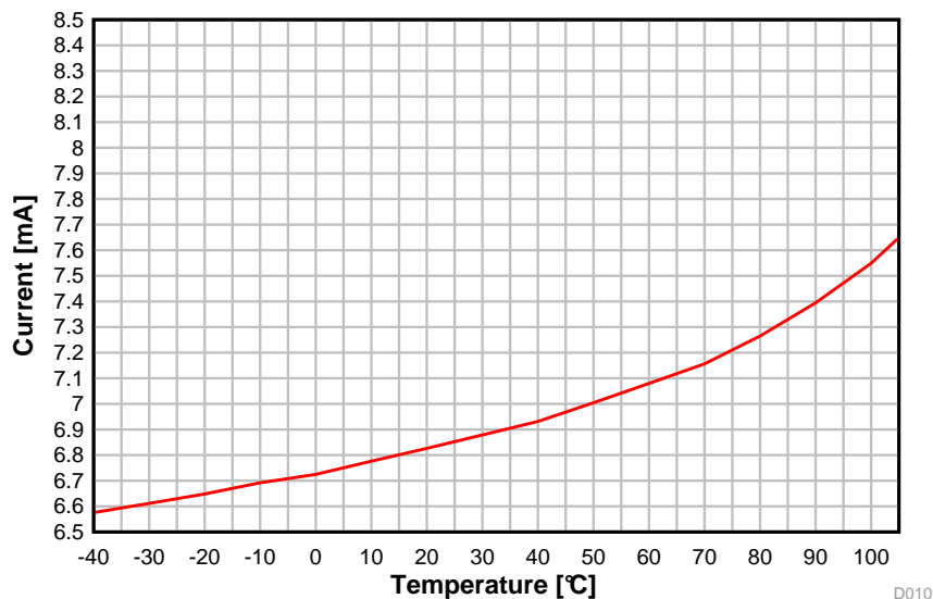
图 5-7. RX Current vs. Temperature (BLE 1 Mbps, 2.44 GHz)
