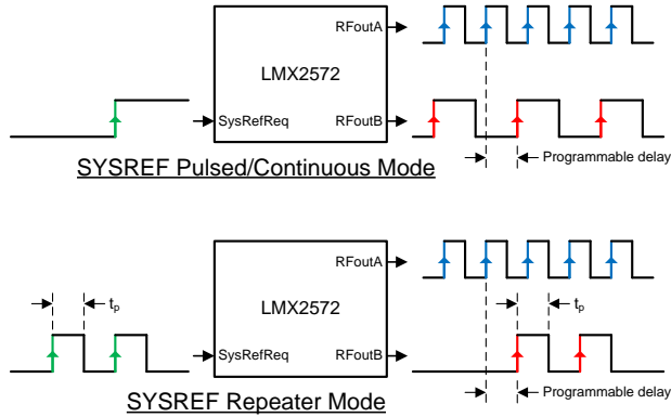
图 35. SYSREF Modes
