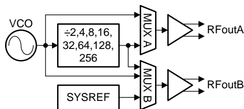
图 32. Channel Divider
