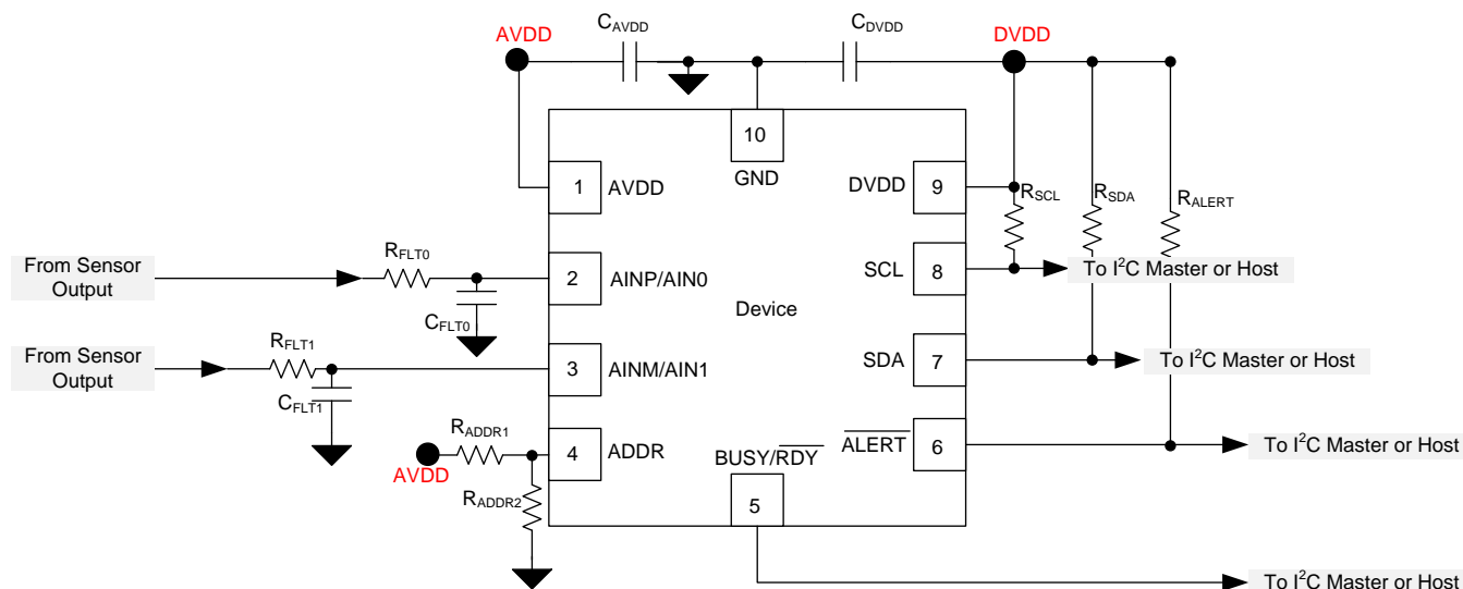
图 123. Example Circuit
