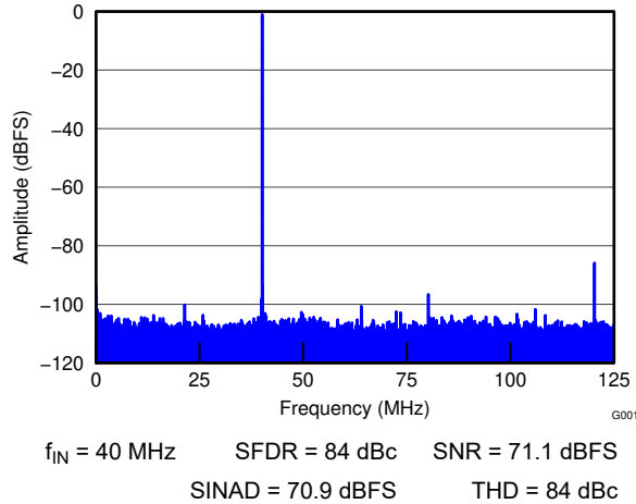
图 6-2. FFT for 40-MHz Input Signal
