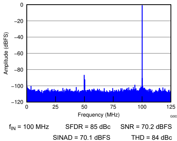
图 6-4. FFT for 100-MHz Input Signal
