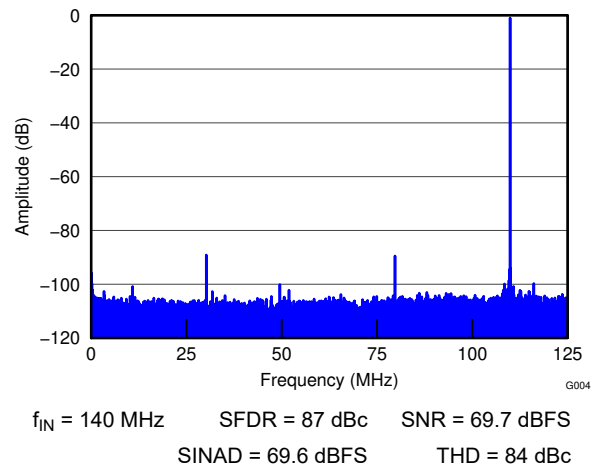
图 6-5. FFT for 140-MHz Input Signal
