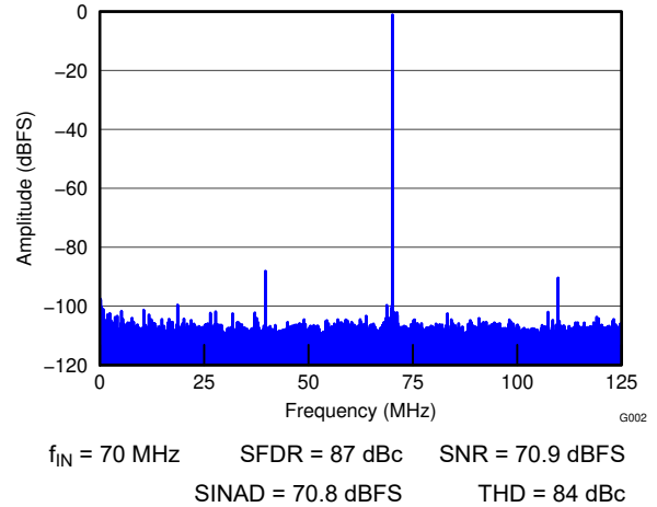
图 6-3. FFT for 70-MHz Input Signal
