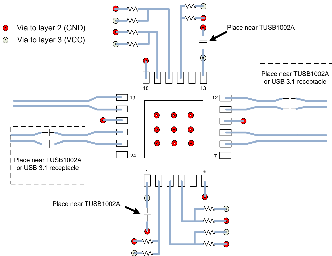
图 25. Example Layout
