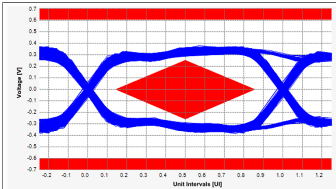
图 23. PCIe Gen1 TX Eye Diagram
