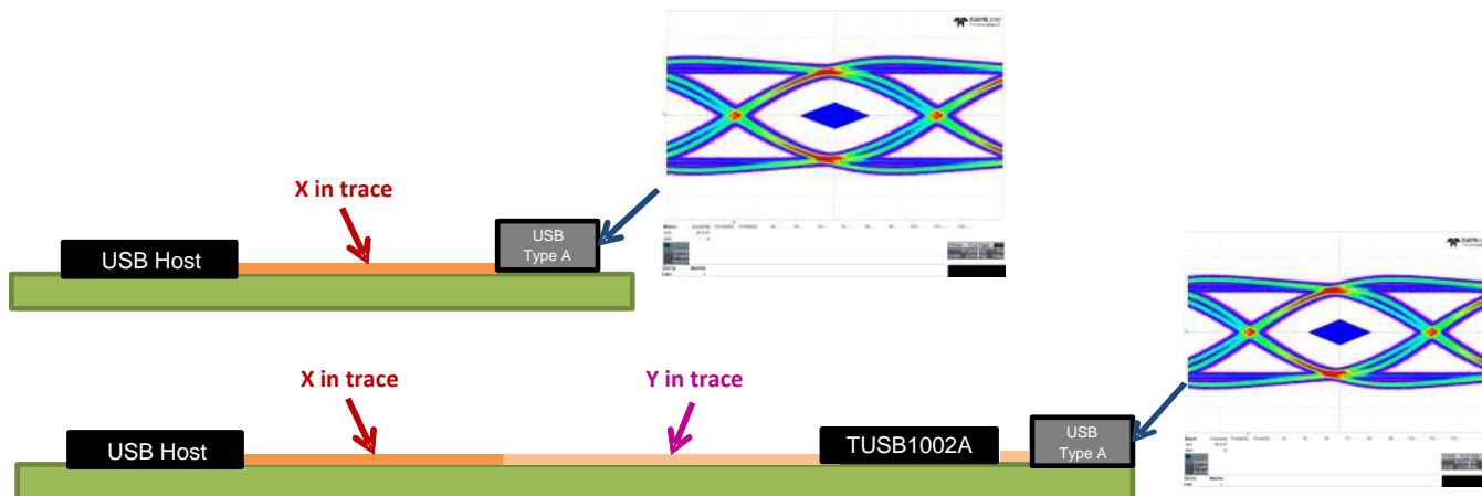
图 16. Linear Equalizer
