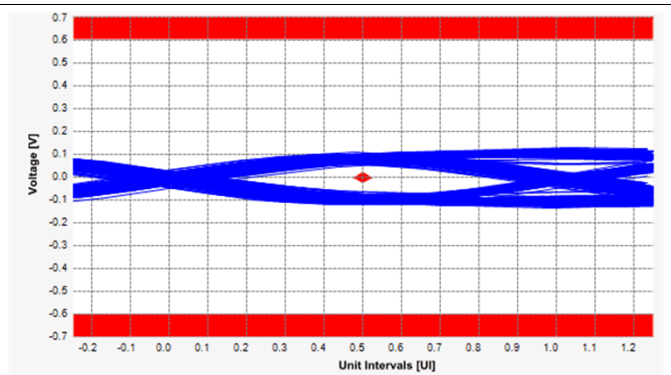
图 24. PCIe Gen3 TX Eye Diagram
