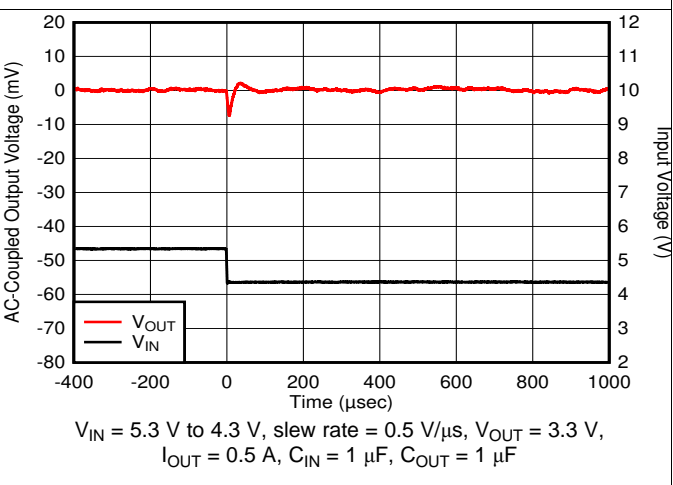
图 30. Line Transient
