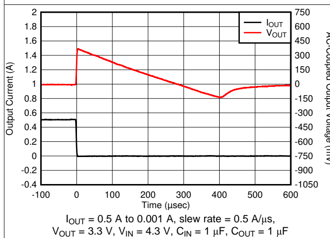
图 29. Load Transient
