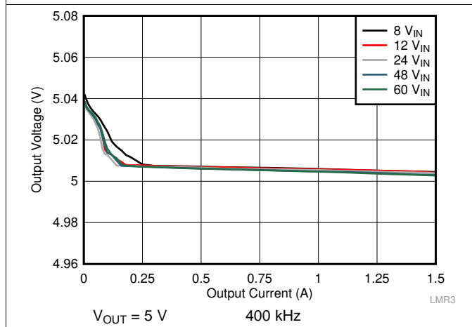
图 24. Load Regulation
