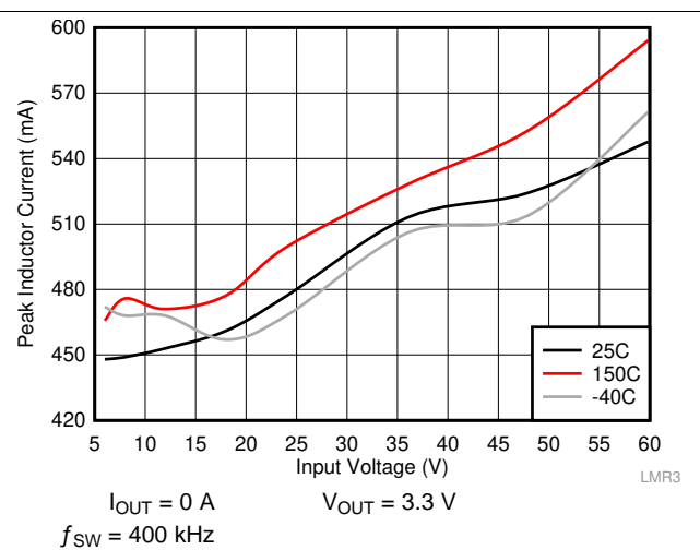
图 6. I PEAK-MIN
