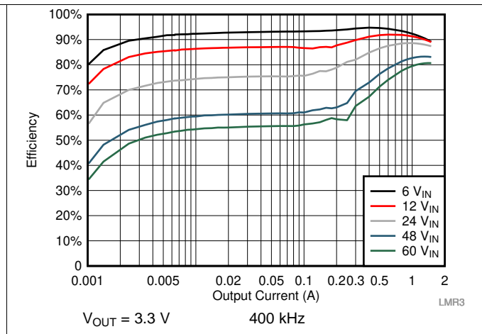
图 23. Efficiency
