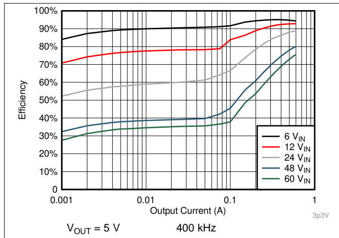
图 22. Efficiency
