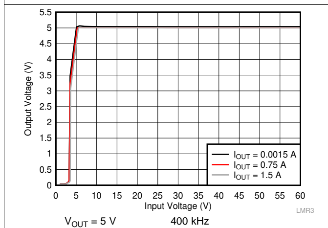
图 26. Line Regulation
