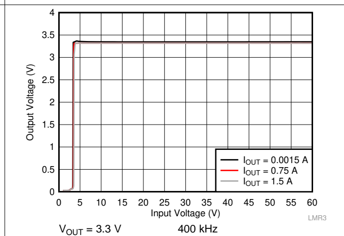
图 27. Line Regulation
