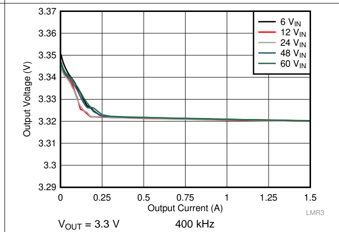
图 25. Load Regulation
