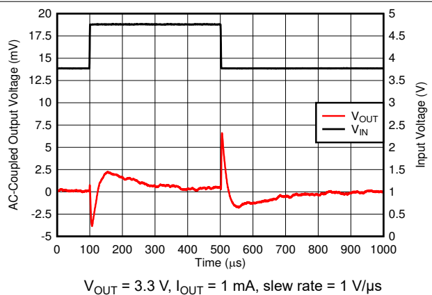
图 6-24. Line Transient
