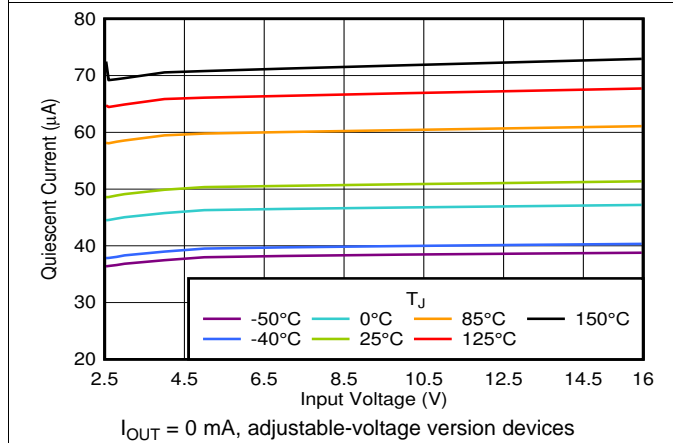
图 5. I_Q vs V_{IN}
