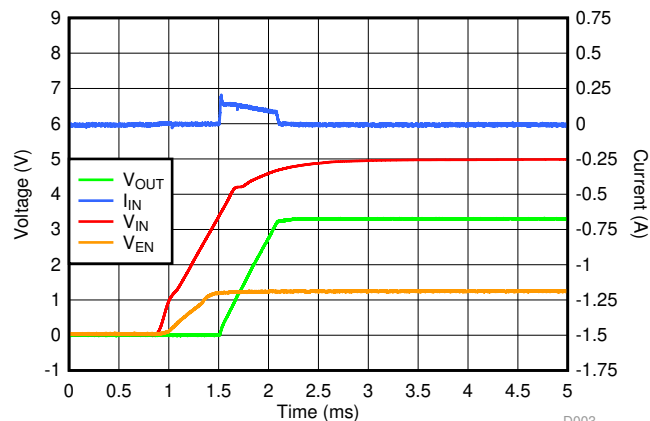
C_{\text{OUT}} 为 22 \mu\text{F} 时减小的浪涌电流
