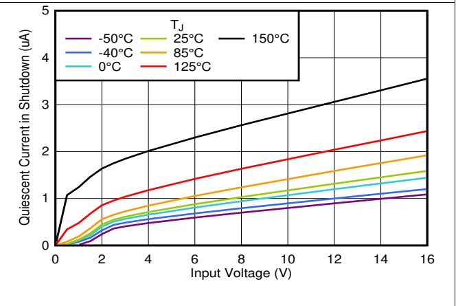
图 4. I_{SHUTDOWN} vs V_{IN}
