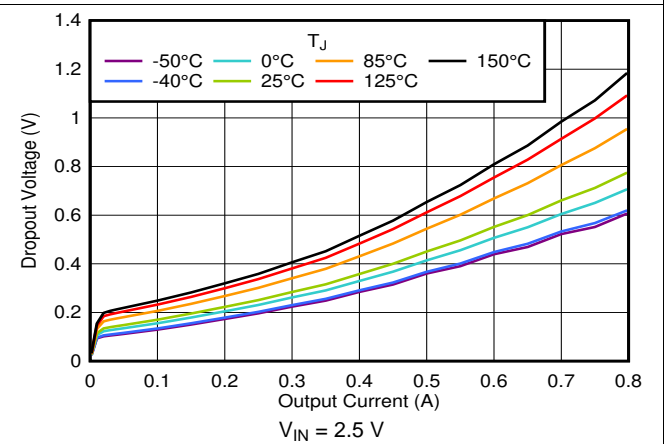
图 18. V_{DO} vs I_{OUT}
