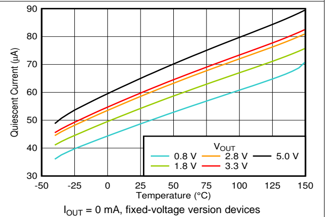
图 6. I_Q vs Temperature
