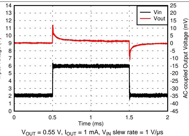
图 18. 0.55-V Line Transient
