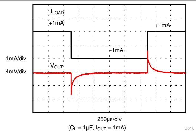
图 7-10. Load Transient
