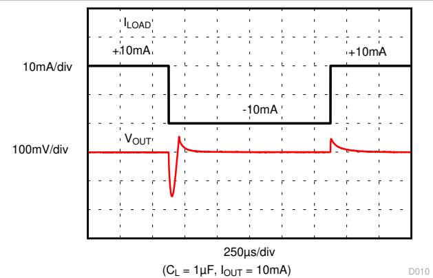
图 7-12. Load Transient
