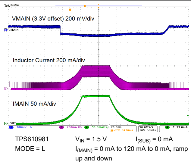
图 9-18. Load Regulation
