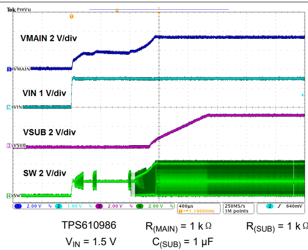
图 9-22. Startup
