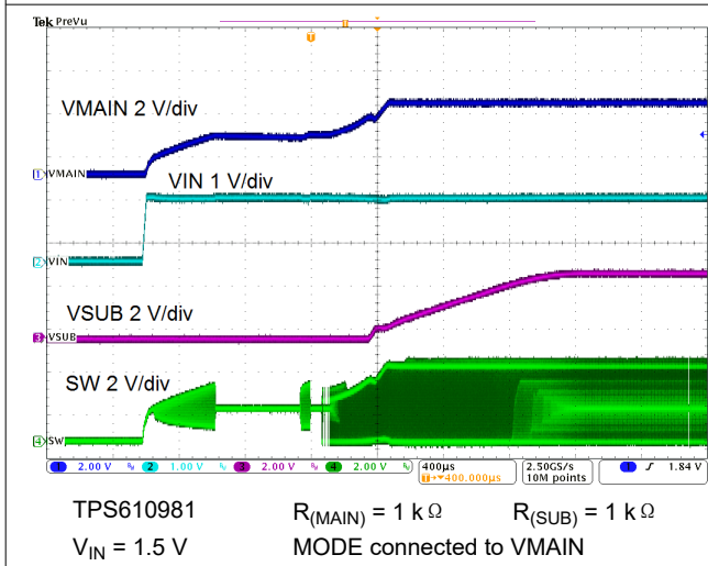
图 9-23. Startup
