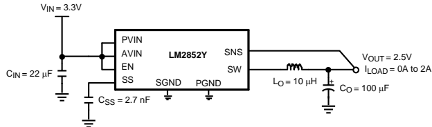
典型应用电路
