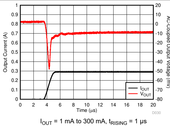
图 6-51. Load Transient
