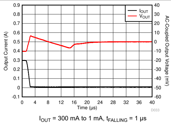
图 6-52. Load Transient
