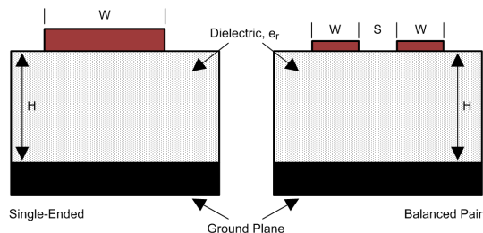
图 11-1. Microstrip Topology
