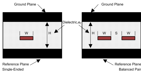
图 11-2. Stripline Topology
