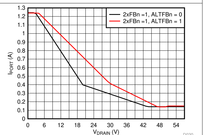
图 30. 2x 模式 (2xFBn = 1) 电流折返与漏极电压间的关系
