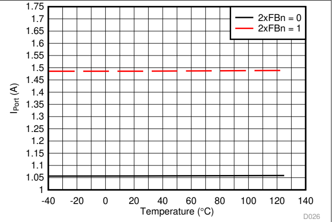
图 26. I_SHORT 阈值与温度间的关系
