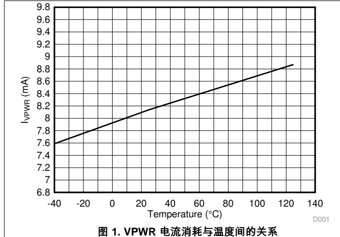
图 1. VPWR 电流消耗与温度间的关系
