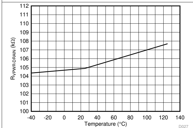
图 27. R_OFF (VPWR 至 DRAIN) 与温度间的关系
