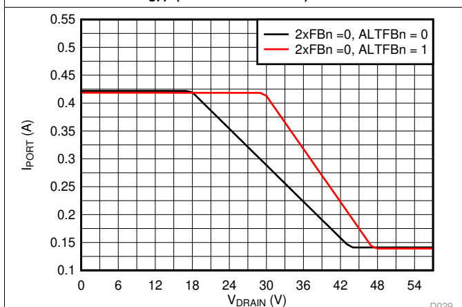
图 29. 1x 模式 (2xFBn = 0) 电流折返与漏极电压间的关系
