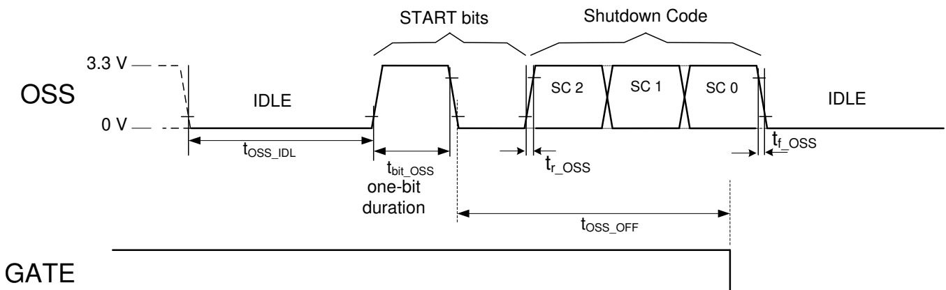
图 38. 如果是较低优先级端口，多位优先级端口将关断
