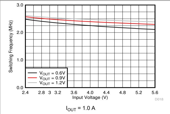
图 9-9. Switching Frequency
