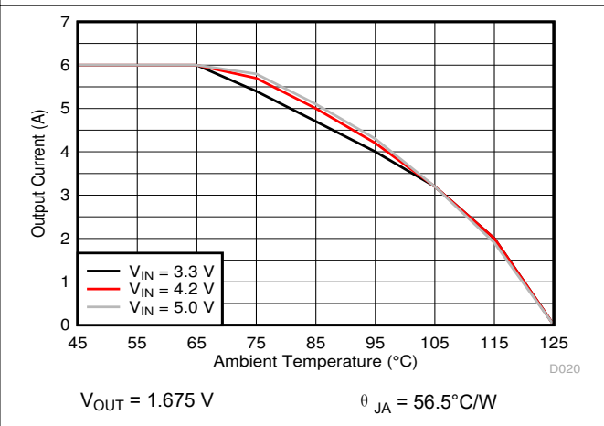
图 9-11. Thermal Derating
