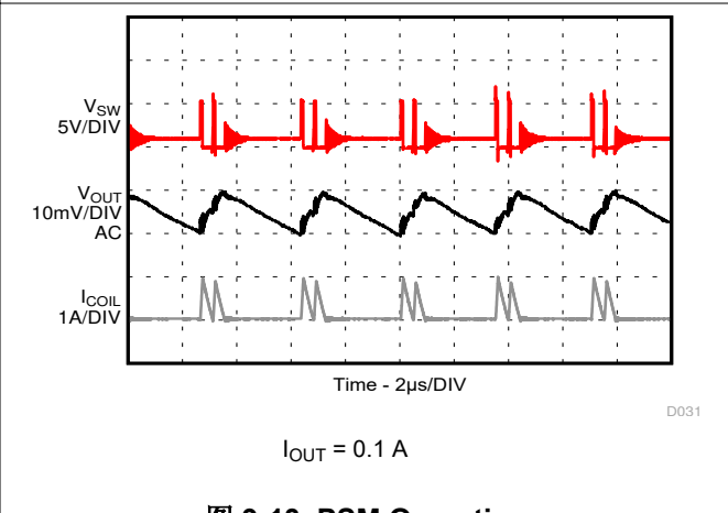
图 9-13. PSM Operation
