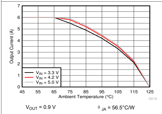
图 9-10. Thermal Derating
