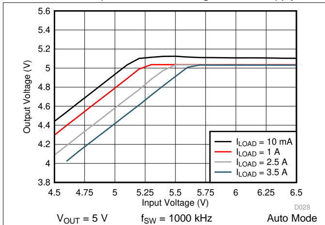
图 53. LM76003-Q1 Dropout Curve
