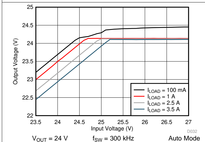
图 57. LM76003-Q1 Dropout Curve
