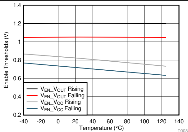
图 8. Enable Threshold
