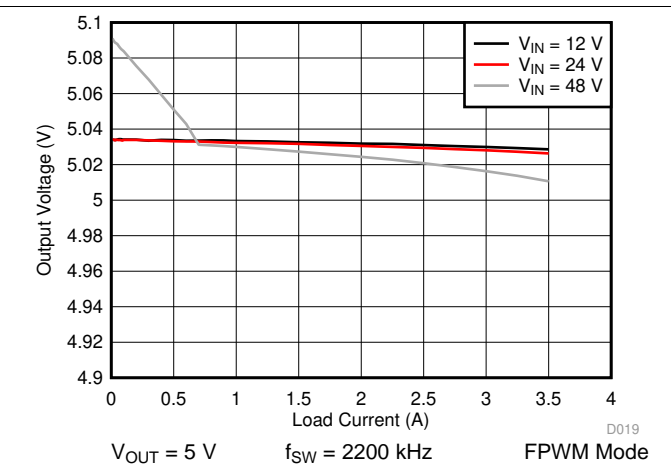
图 44. LM76003-Q1 Load and Line Regulation
