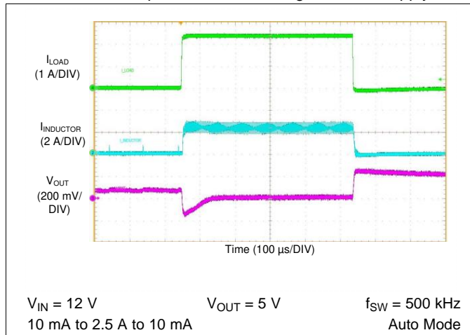
图 83. LM76002-Q1 Load Transient
