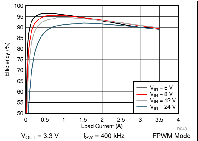
图 24. LM76003-Q1 Efficiency
