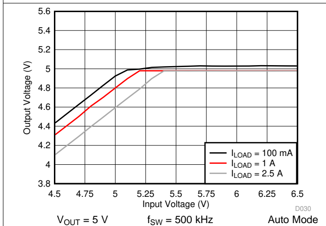
图 55. LM76002-Q1 Dropout Curve
