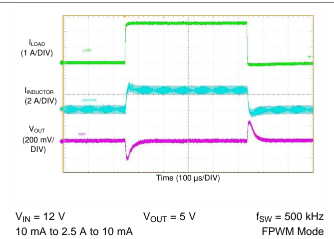
图 84. LM76002-Q1 Load Transient
