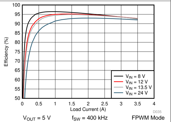
图 26. LM76003-Q1 Efficiency
