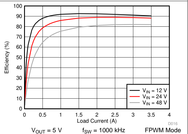
图 28. LM76003-Q1 Efficiency
