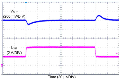
图 10-23. LM62440-Q1 Load Transient
