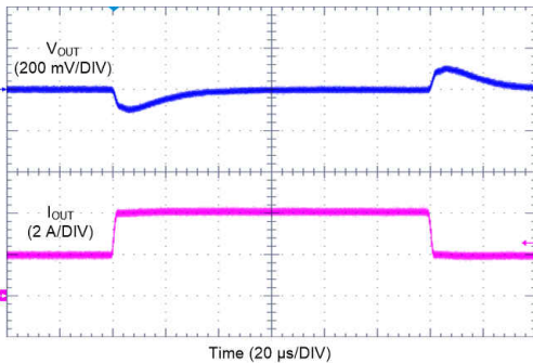
图 10-25. LM62440-Q1 Load Transient
