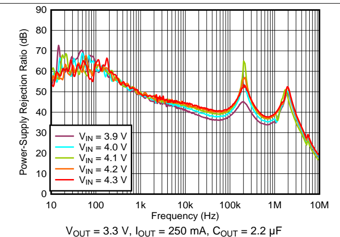
图 28. PSRR vs Frequency and V_{IN}
