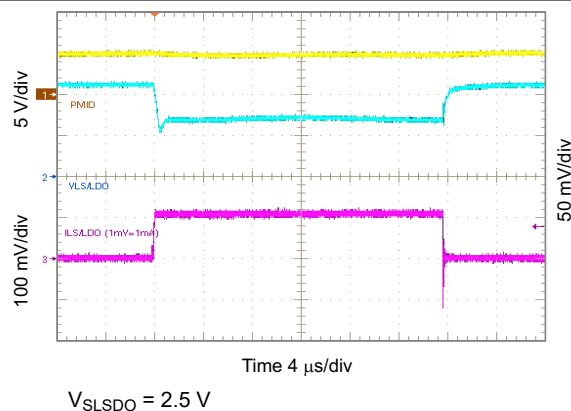
图 10-53. 2.5 V_{LSLDO} Load Transient, 0 to 100 mA
