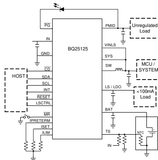
简化版原理图
