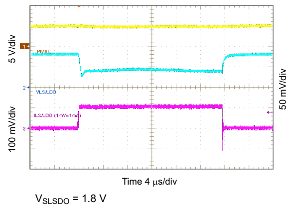
图 10-52. 1.8 V_{LSLDO} Load Transient, 0 to 100 mA
