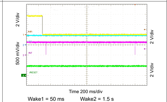
图 10-62. Show \overline{MR} Timing
