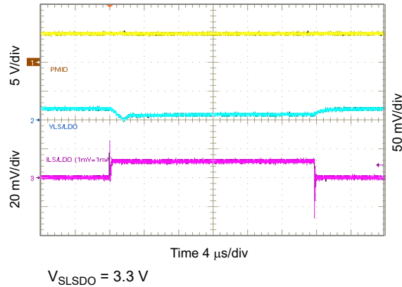
图 10-49. 3.3 V_{LSLDO} Load Transient, 0 to 10 mA
