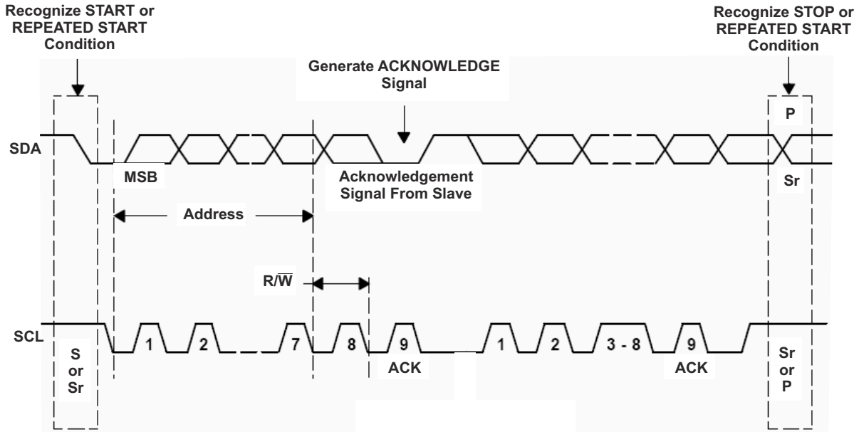
图 9-10. Bus Protocol
