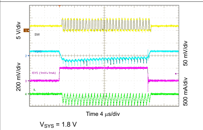
图 10-37. 1.8 V_{SYS} Load Transient, 0 to 200 mA
