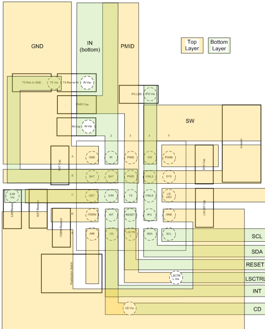
图 12-1. BQ25125 Layout
