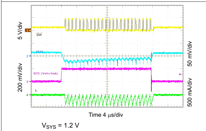
图 10-36. 1.2 V_{SYS} Load Transient, 0 to 200 mA
