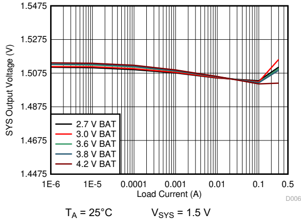
图 10-14. 1.5 V sys Load Regulation
