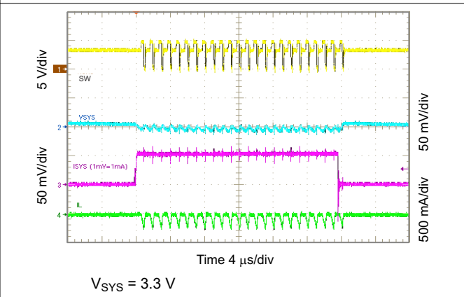
图 10-35. 3.3 V_{SYS} Load Transient, 0 to 50 mA
