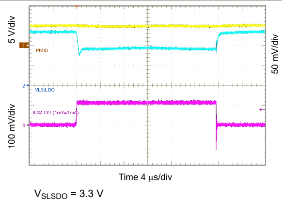
图 10-54. 3.3 V_{LSLDO} Load Transient, 0 to 100 mA
