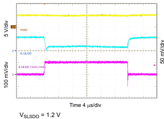
图 10-51. 1.2 V_{LSLDO} Load Transient, 0 to 100 mA
