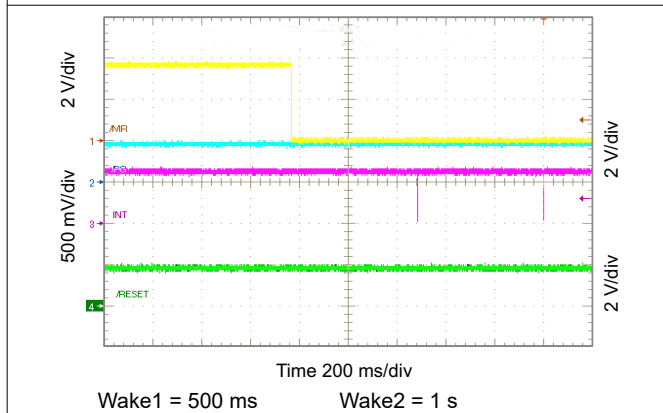
图 10-61. Show \overline{MR} Timing
