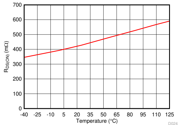
图 8-6. Blocking FET R DS(ON) vs Temperature
