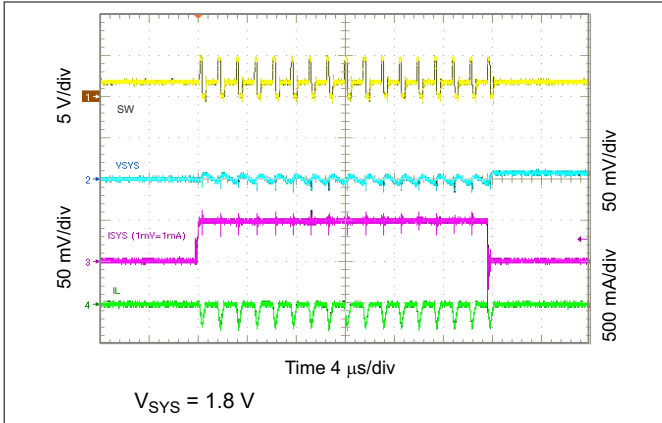
图 10-32. 1.8 V_{SYS} Load Transient, 0 to 50 mA
