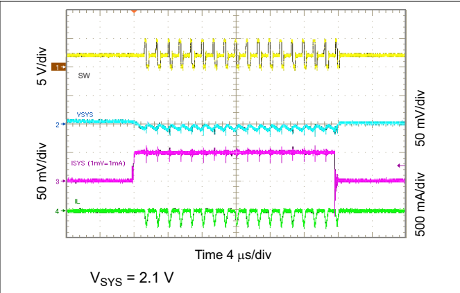
图 10-33. 2.1 V_{SYS} Load Transient, 0 to 50 mA
