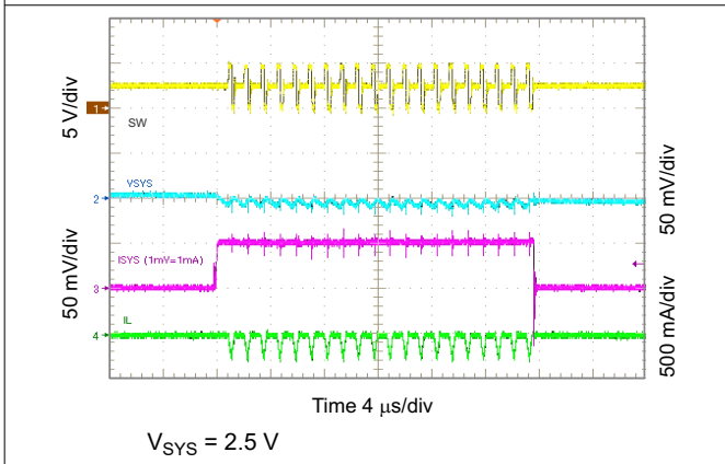
图 10-34. 2.5 V_{SYS} Load Transient, 0 to 50 mA
