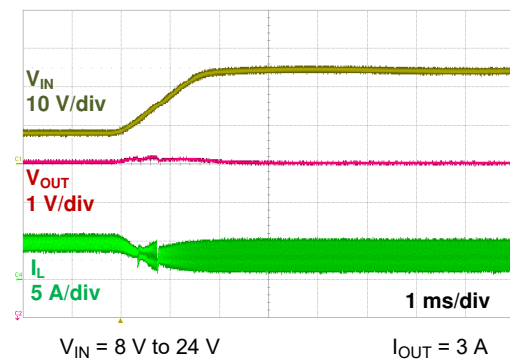
图 6-18. Line Transient
