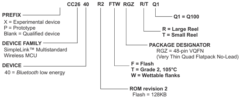
图 11-1. Device Nomenclature
