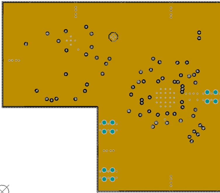
图 95. Ground Layer 1
