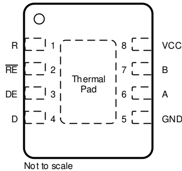
图 5-2. DRB (VSON), 8 引脚封装, 顶视图
