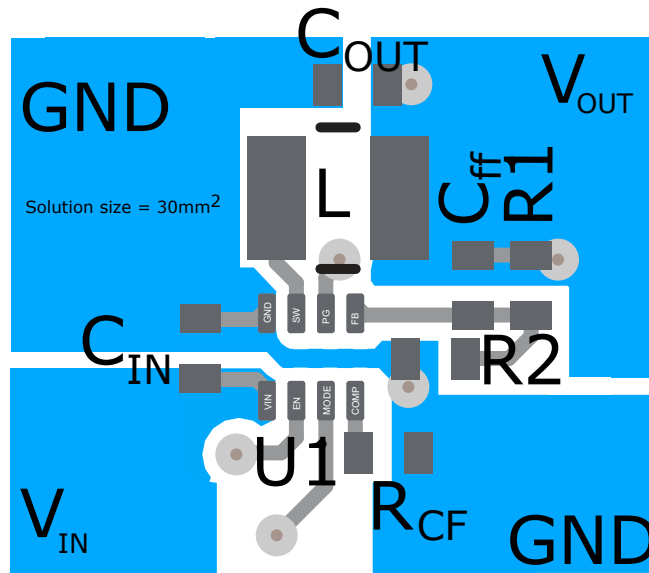
图 12-1. Example Layout
