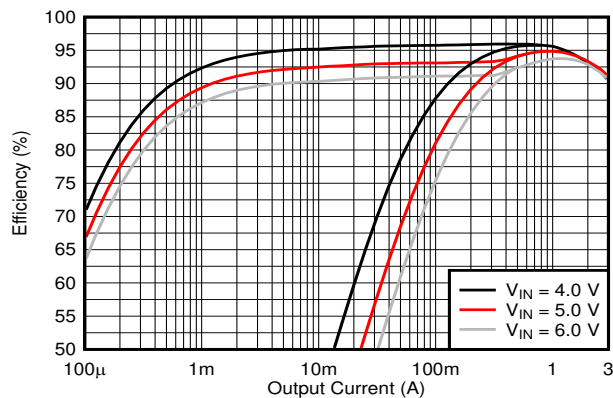
效率与 I_{OUT} 间的关系， V_{OUT} = 3.3\text{V}
