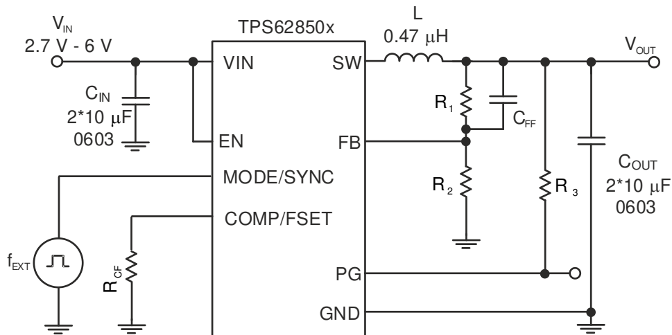
图 10-57. Schematic using External Synchronization
