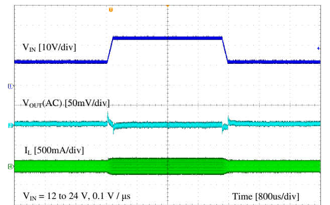
图 9-8. Line Transient
