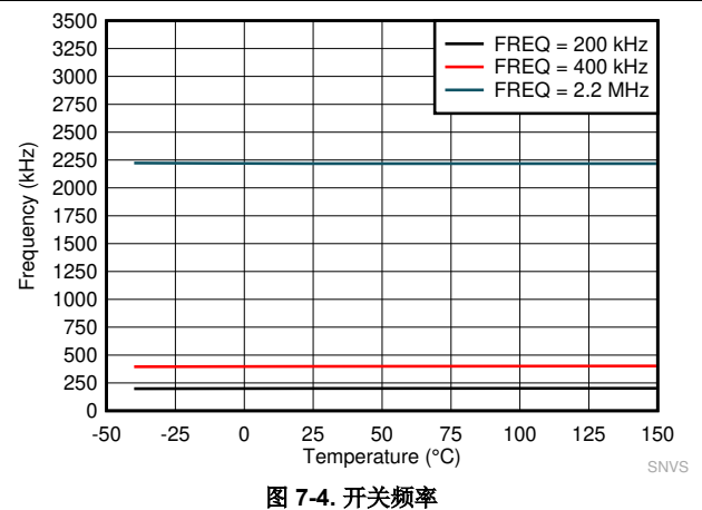
图 7-4. 开关频率
