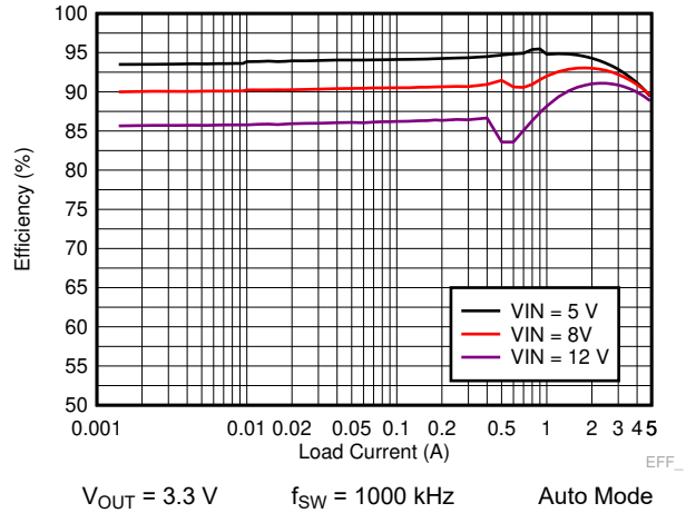
图 9-10. LM73605-Q1 Efficiency
