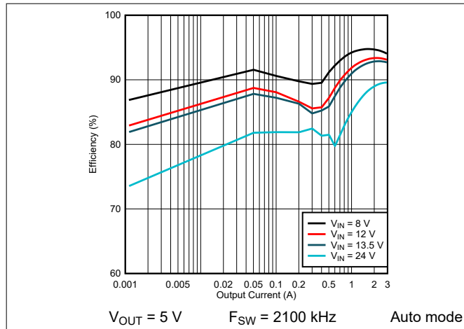
图 9-10. LM61430-Q1 Efficiency
