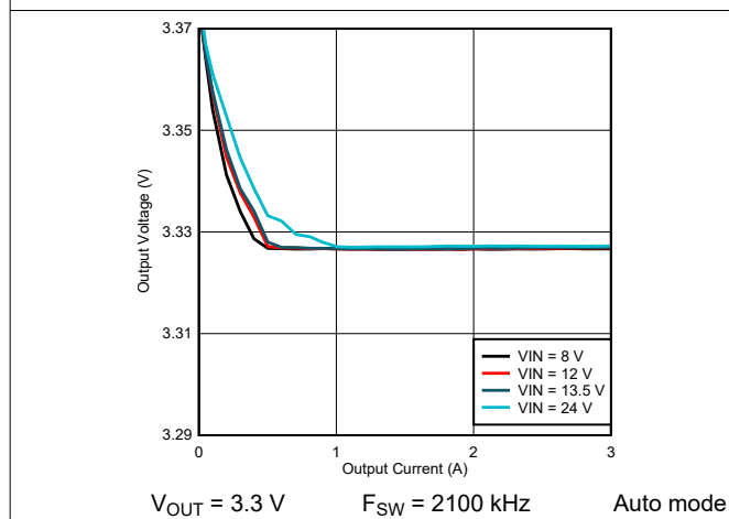
图 9-14. LM614630-Q1 Load and Line Regulation
