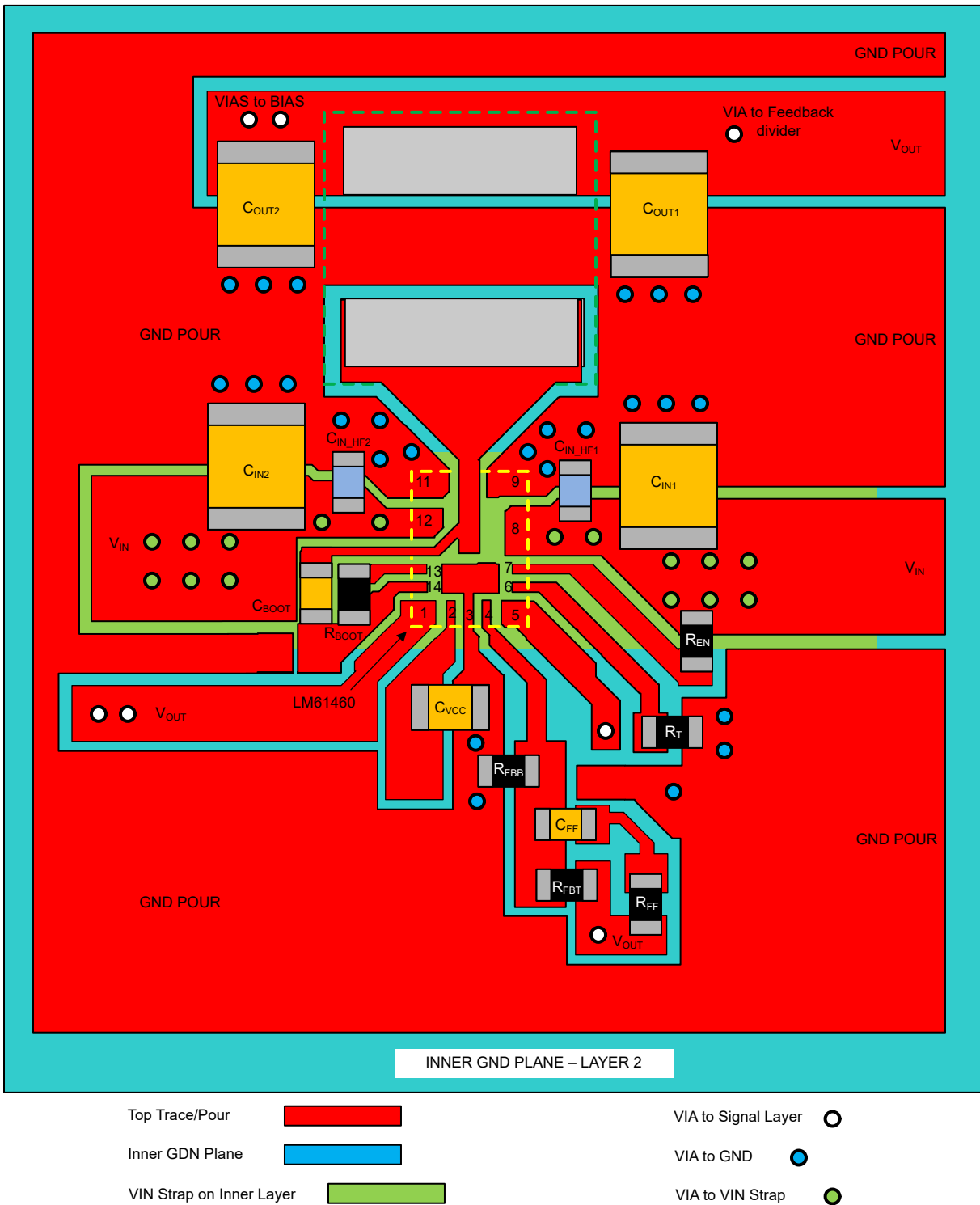
图 11-2. Layout Example
