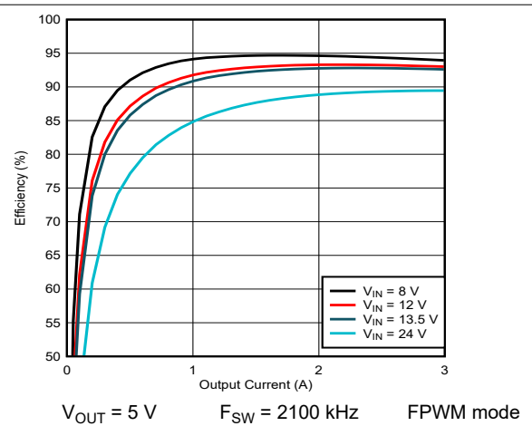
图 9-11. LM61430-Q1 Efficiency
