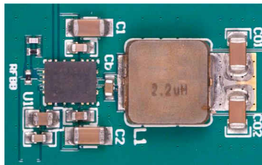
典型车用布局 (22mm x 12.5mm)
