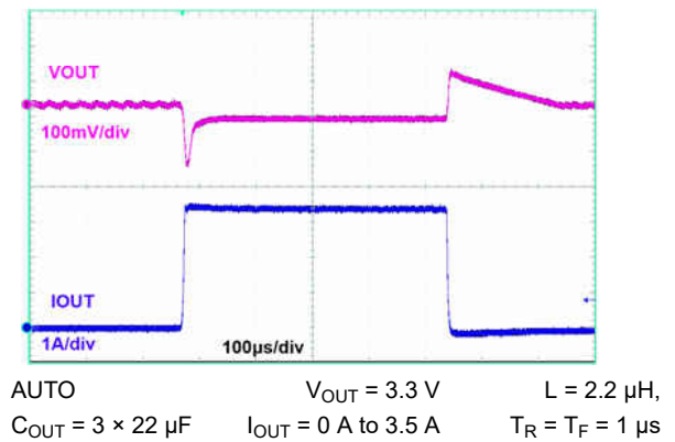
图 9-30. Load Transient
