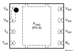
俯视图
