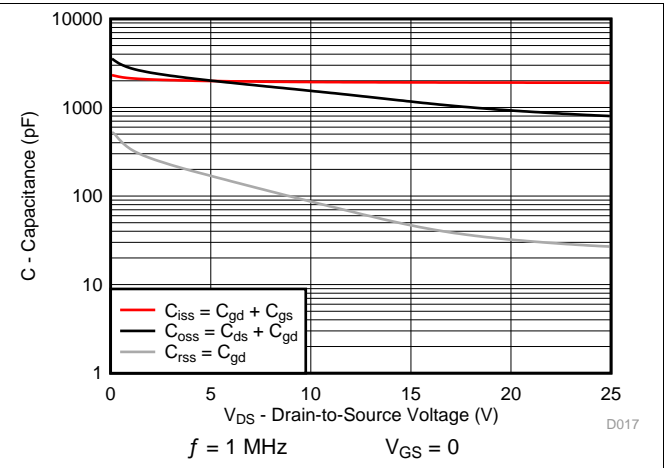
图 15. Sync MOSFET Capacitance
