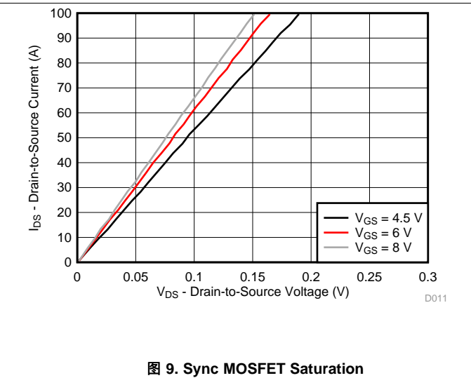
图 9. Sync MOSFET Saturation
