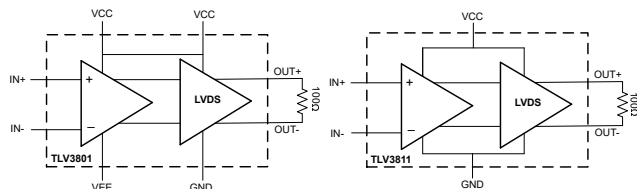
功能方框图
