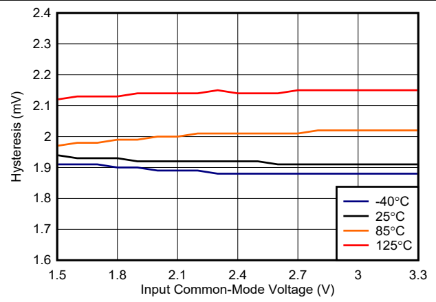
图 6-6. Hysteresis vs. Common-Mode, 3.3 V
