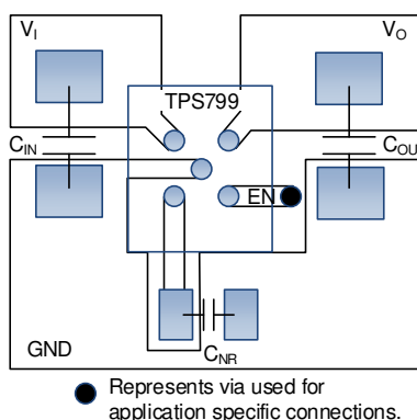
图 10-1. Layout Example
