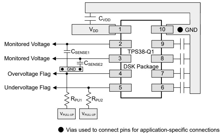
图 12-1. TPS38-Q1 DSK Package Recommended Layout
