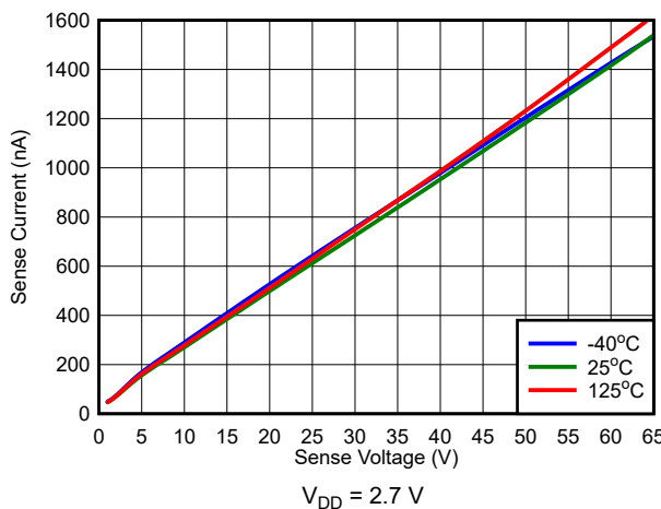
图 7-7. V_{SENSE} vs I_{SENSE}
