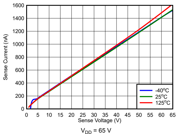
图 7-8. V_{SENSE} vs I_{SENSE}
