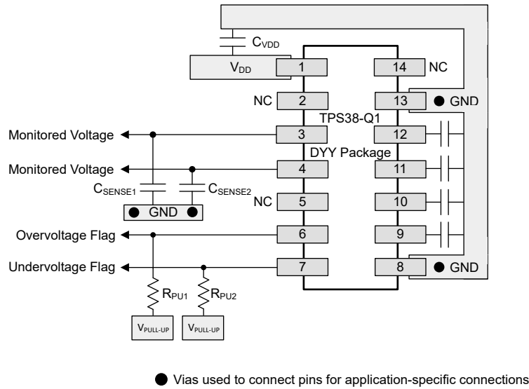
图 12-2. TPS38-Q1 DYY Package Recommended Layout
