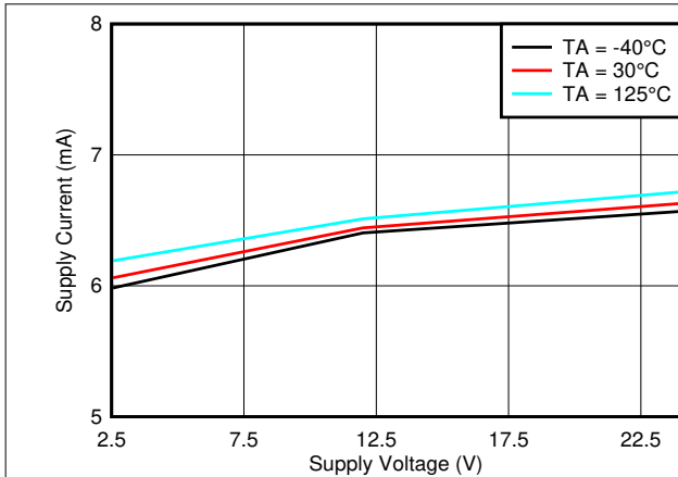
图 7-75. 电源电流与 V_{CC}
