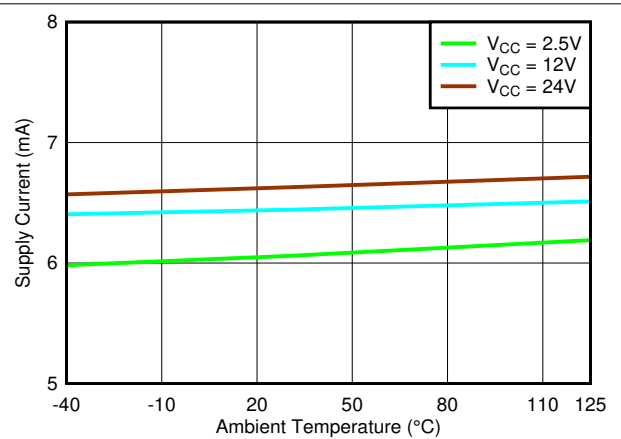
图 7-76. 电源电流与温度间的关系
