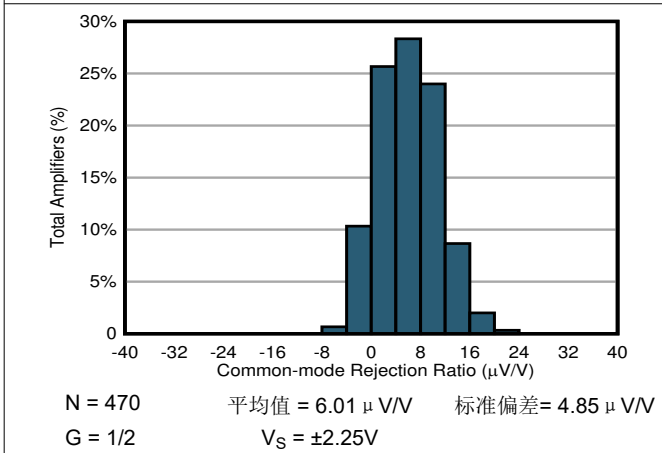
图 7-15. 典型 CMRR 分布
