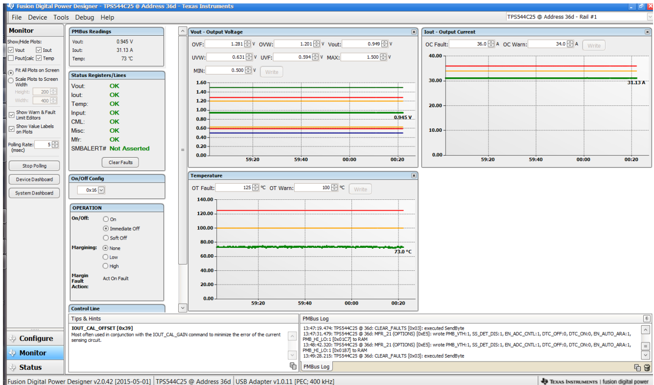
图 57. 使用 Fusion Digital Power Designer 进行器件监控
