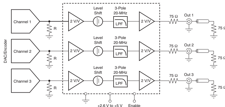
简化的应用电路
